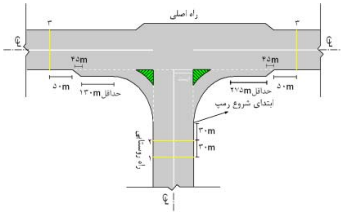
شکل ۵- ساماندهی و ایمن سازی در تقاطع های راه روستایی به اصلی
