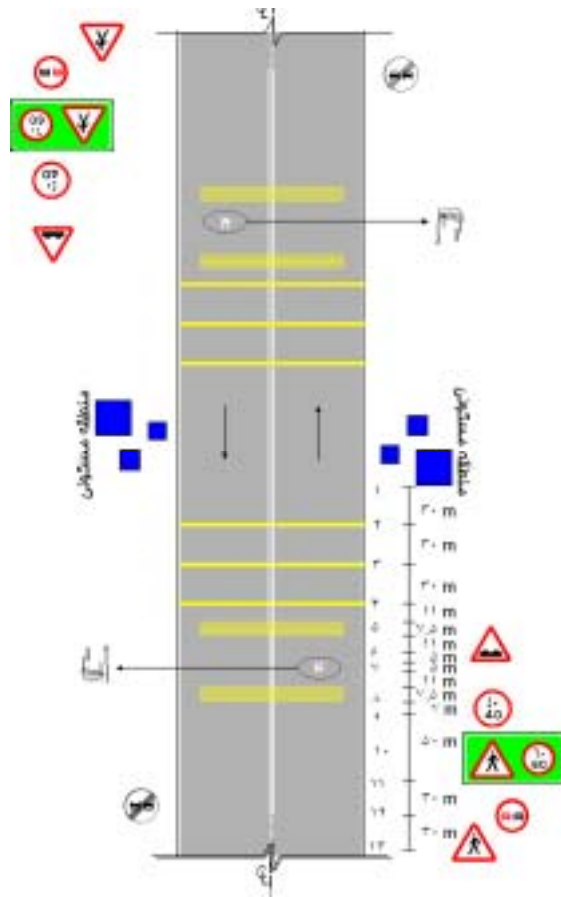
شکل ۹- ایمن سازی مناطق مسکونی در راههای فرعی با دید کافی
