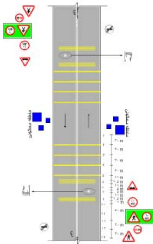
شکل ۱۰- ایمن سازی مناطق مسکونی در راههای فرعی با محدودیت دید
